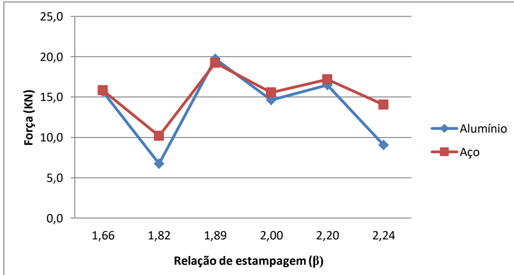
Figura 7- Valores máximos de força, em KN, para cada um dos valores de relação de estampagem ( \beta ).
