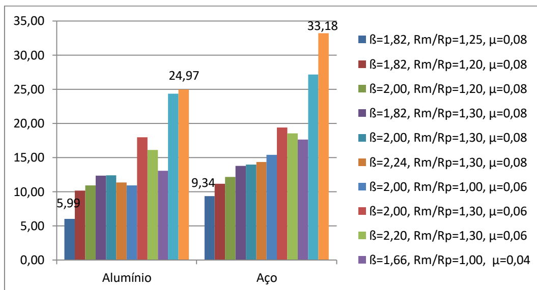
Figura 10-Comparação geral entre alumínio e aço com relação a altura de embutimento antes de haver a ruptura. Cada uma das barras tem um valor para os parâmetros \beta , R_m/R_p , \mu .
